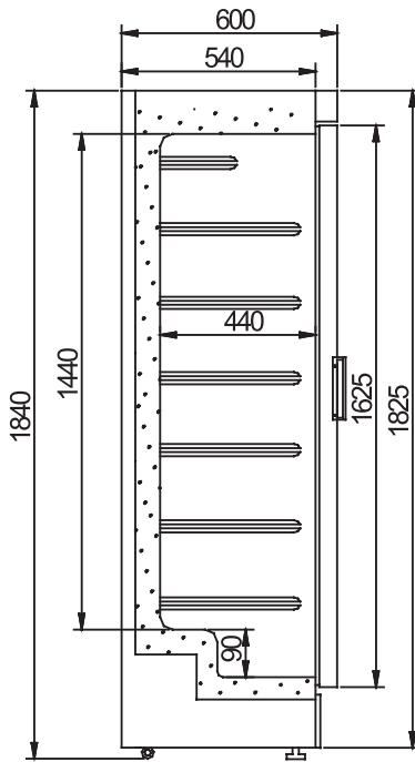
UDD 370 DTKL
