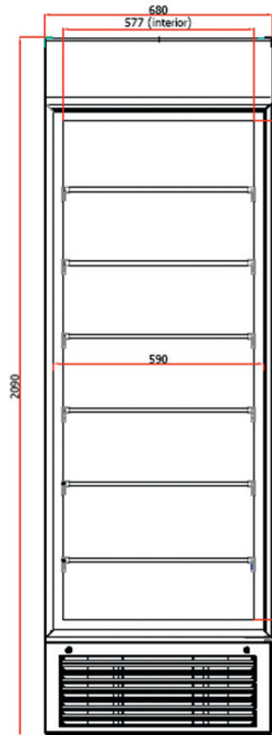
UDD 440 DTKL
