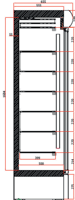
UDD 440 DTKLB
