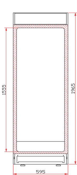
UDD 370 DTKL
