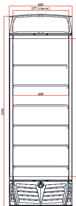
UDD 440 DTKLB
